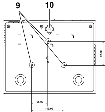
底視圖
